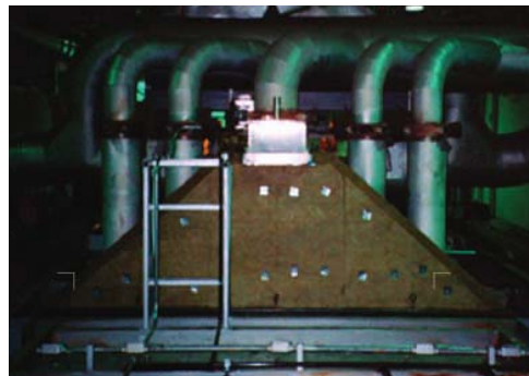
Float Glass Annealing Lehr
