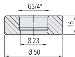
Brida de soldo para G3/4" membrana frontal (1.4301) N.º pedido C27805
